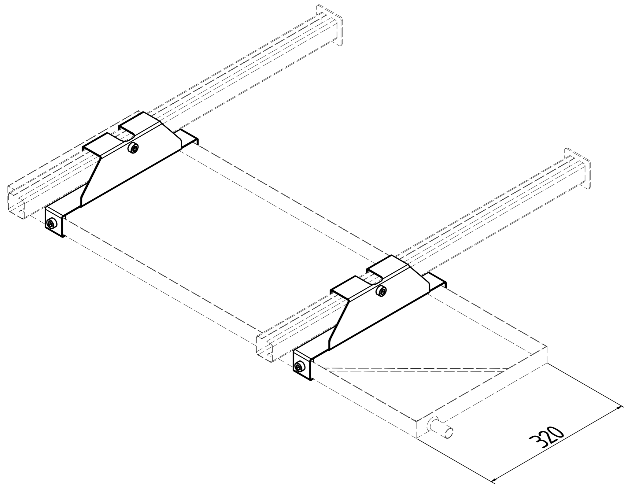
Wannenhalter für Wandkonsolen
